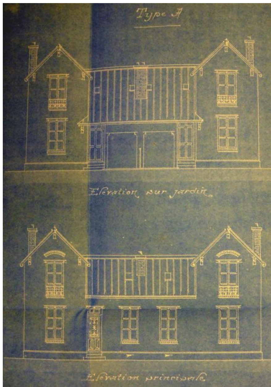
Élévation d'une maison de type A, 1904. (Archives municipales et communautaires d'Orléans, 5 J 130).
