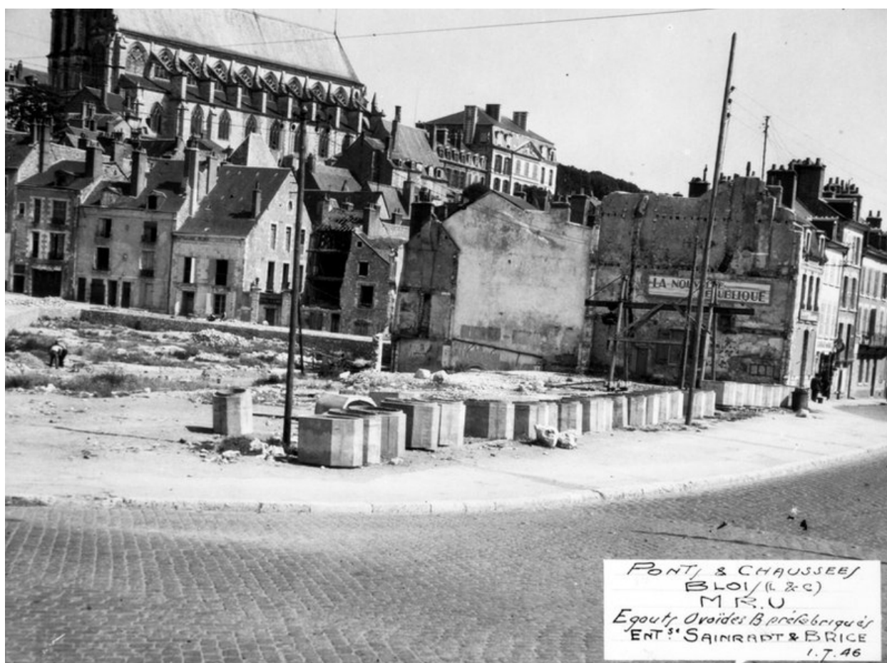
Vue du chantier. Egouts ovoïdes préfabriqués. 1-07-1946. (Archives départementales de Loir-et-Cher, Blois, 1029 W 89).
