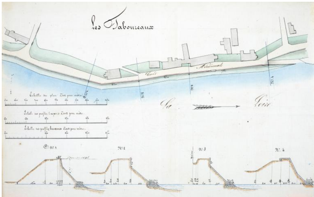
Plan de la Loire aux Taboureaux dressé par l'ingénieur ordinaire Cormier, 6 juin 1850. (archives départementales d'Indre-et-Loire, S 2039).
