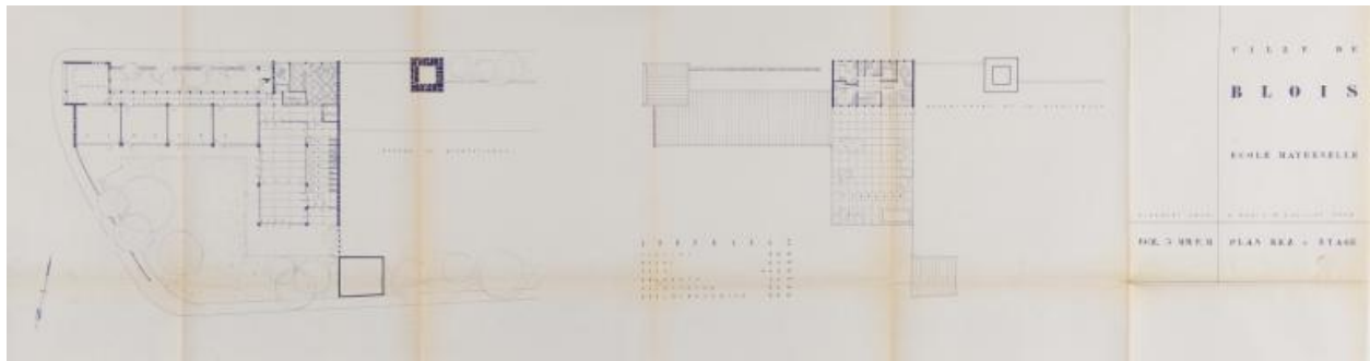
Projet d'école maternelle, plans du rez-de-chaussée et de l'étage par A. Aubert, 07-1954. (Fonds A. Aubert. SIAF/ Cité de l'architecture et du Patrimoine / Archives d'architecture du XXe siècle, 072 IFA : 119).
